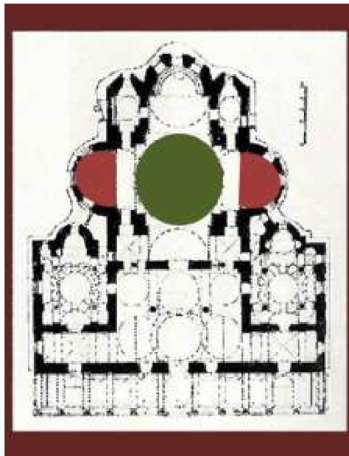
▲ План собора Великой Лавры, Афон
